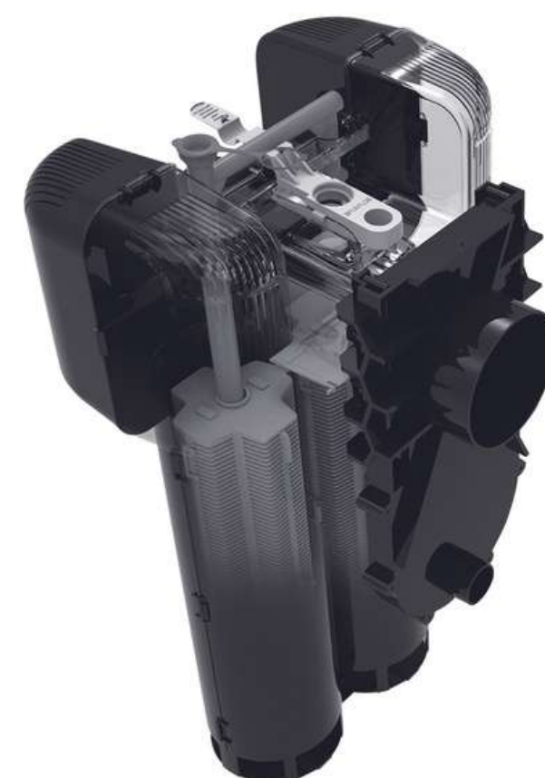
Vue en coupe du préfiltre PF 17
